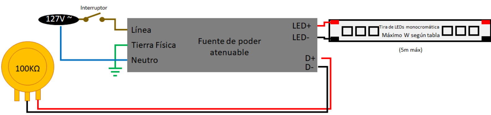
Diagrama para potenciómetro:
