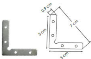
COPLE90PA1911 Conector 90° para perfiles de aluminio serie PA1911, incluye 2 tornillos
