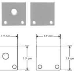
TAPLAT1911G Kit de 2 tapas laterales de plástico para perfil PA1911G
