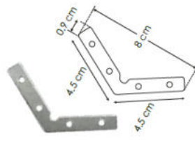
COPLE120PA1911 Conector 120° para perfiles de aluminio serie PA1911, incluye 2 tornillos
