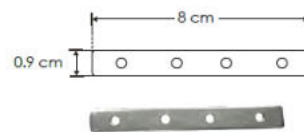
COPLE180PA1911 Conector 180° para perfiles de aluminio serie PA1911, incluye 2 tornillos
