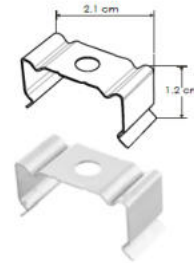
GRAPA1911G Kit de 2 grapas de sujeción para perfil PA1911G
