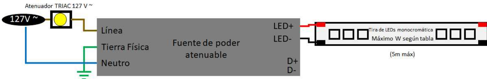
Diagrama para atenuador (Dimmer) tipo TRIAC:
